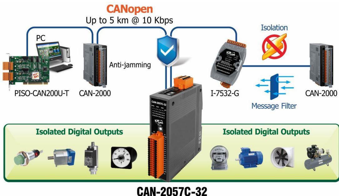
圖 1-2 應用架構
