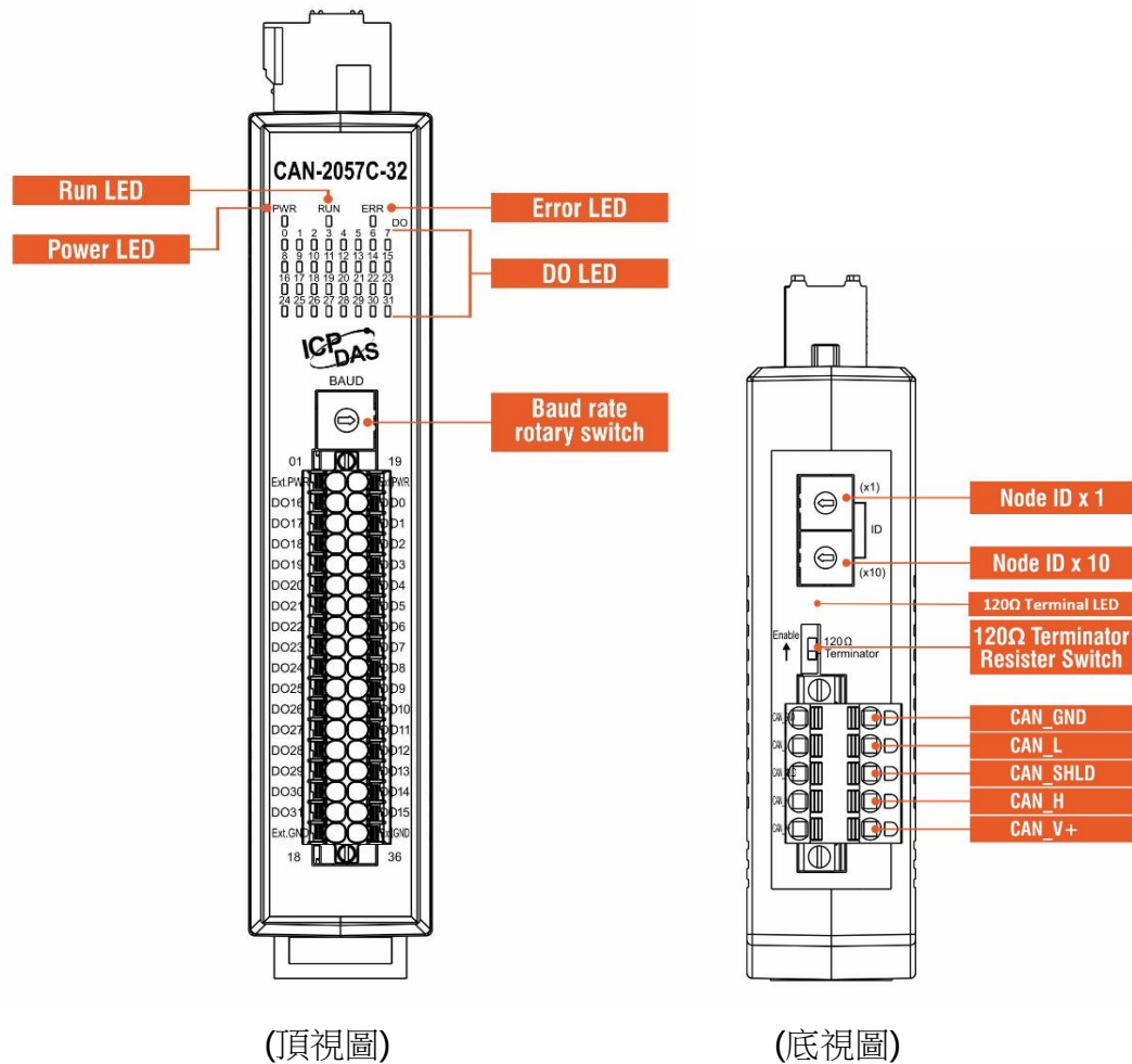
圖 2-1 CAN-2057C-32 LED 規劃圖、端子與旋鈕開關
