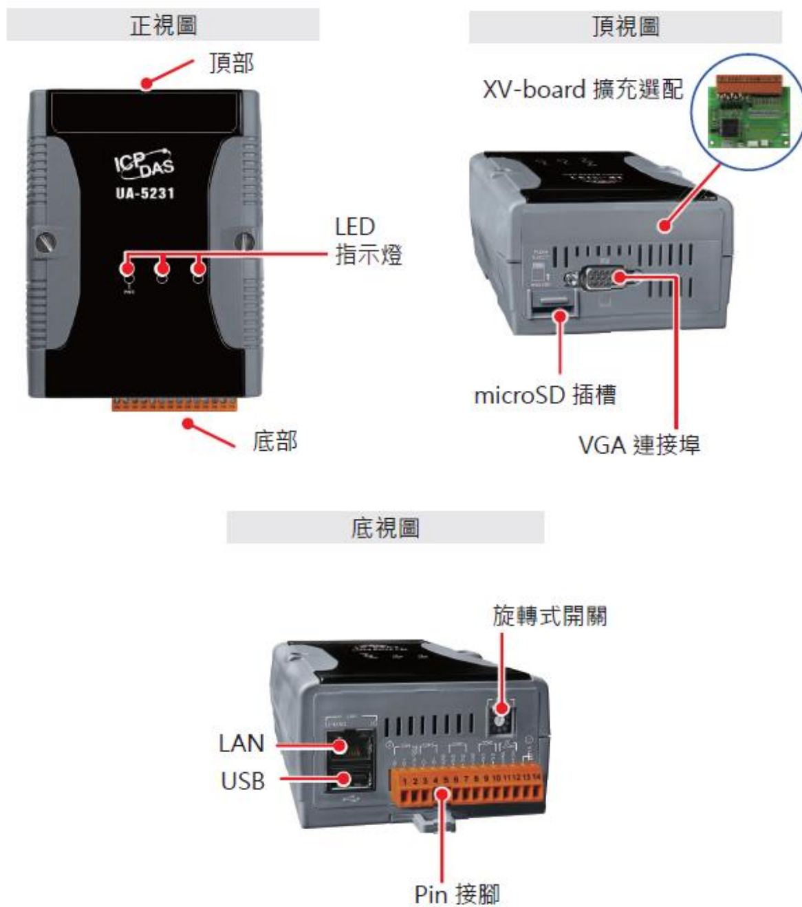
圖 2) 機構圖 UA-5231
