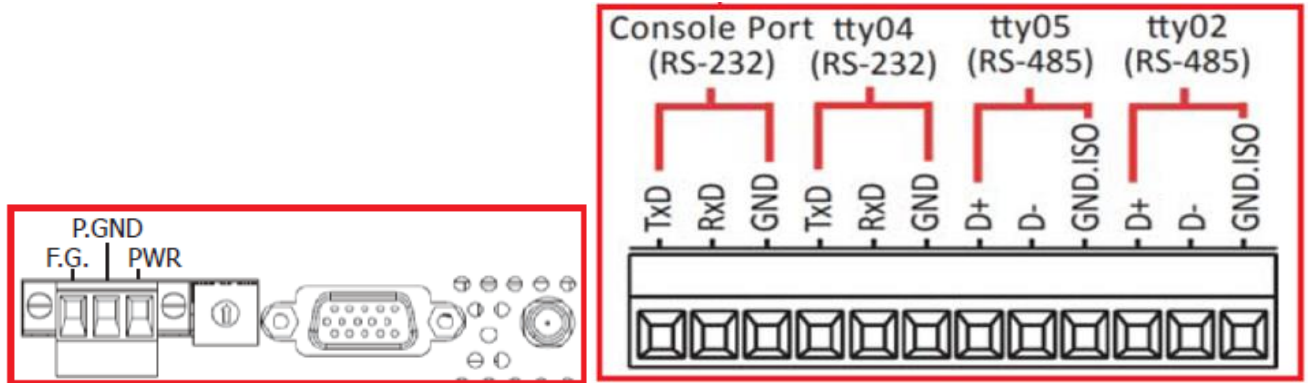
圖 6) 接腳圖 UA-2200 系列
