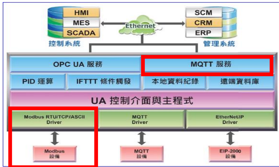
圖 178) MQTT 和 Modbus RTU/ASCII 轉換功能示意圖
