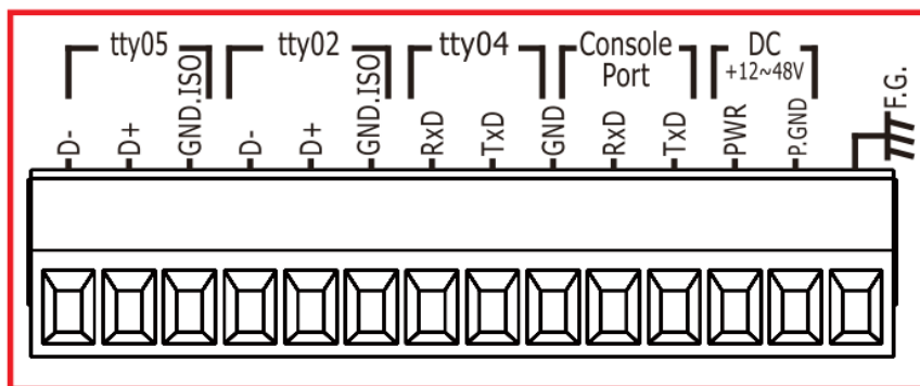
圖 7) 接腳圖 UA-5200 系列-1
