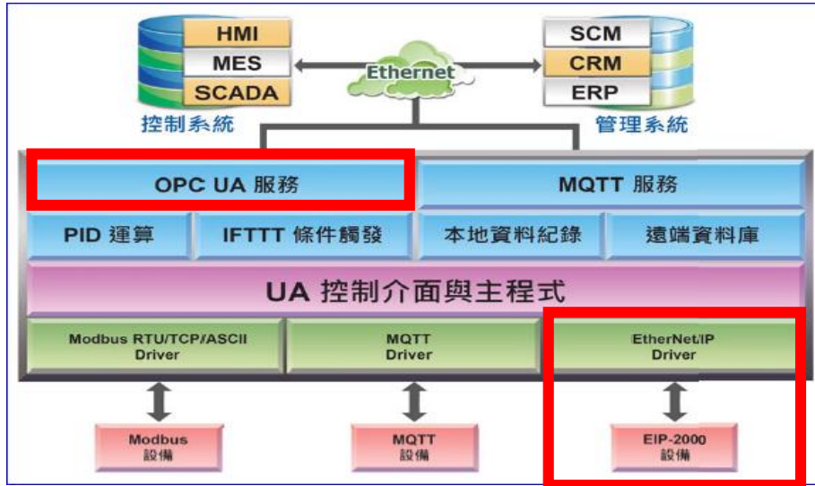
圖 169) OPC UA 和 EtherNet/IP 轉換功能示意圖
