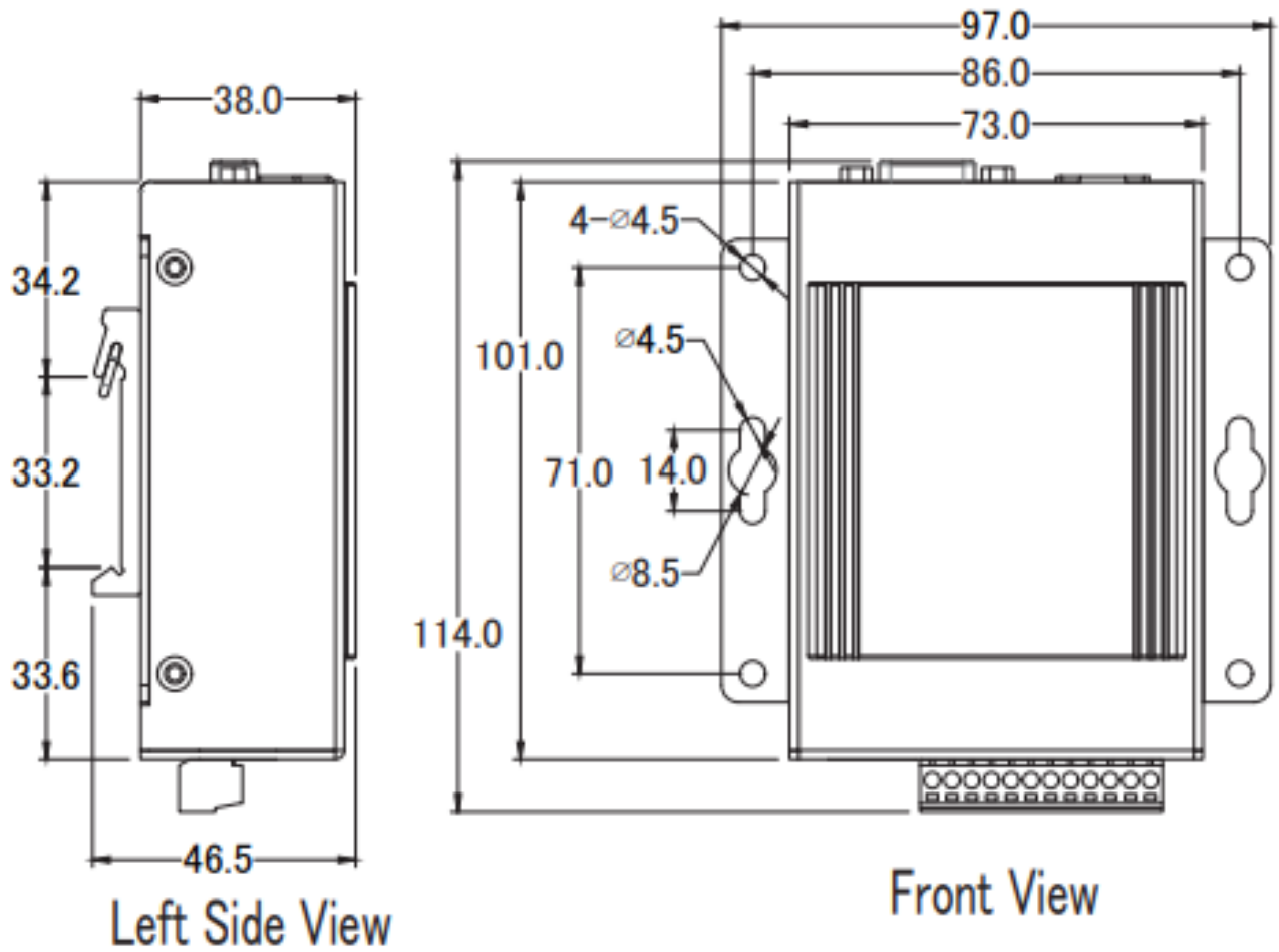
圖 13) 尺寸圖 UA-7231M
