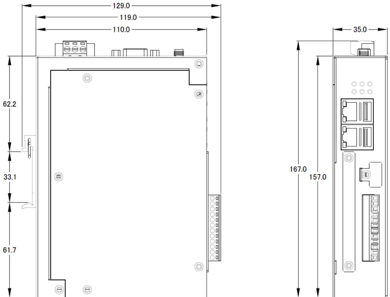
圖 11) 尺寸圖 UA-2200 系列
