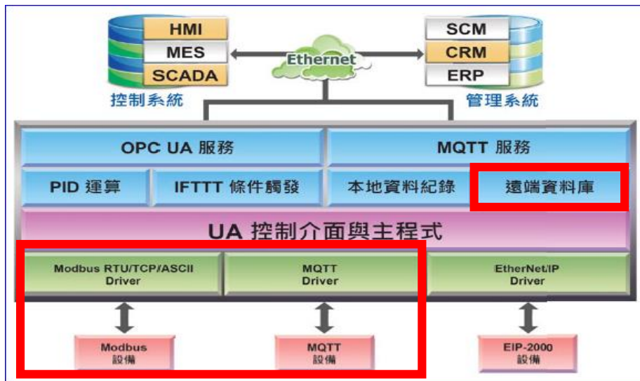
圖 255) MySQL/MariaDB 遠端資料庫功能示意圖
