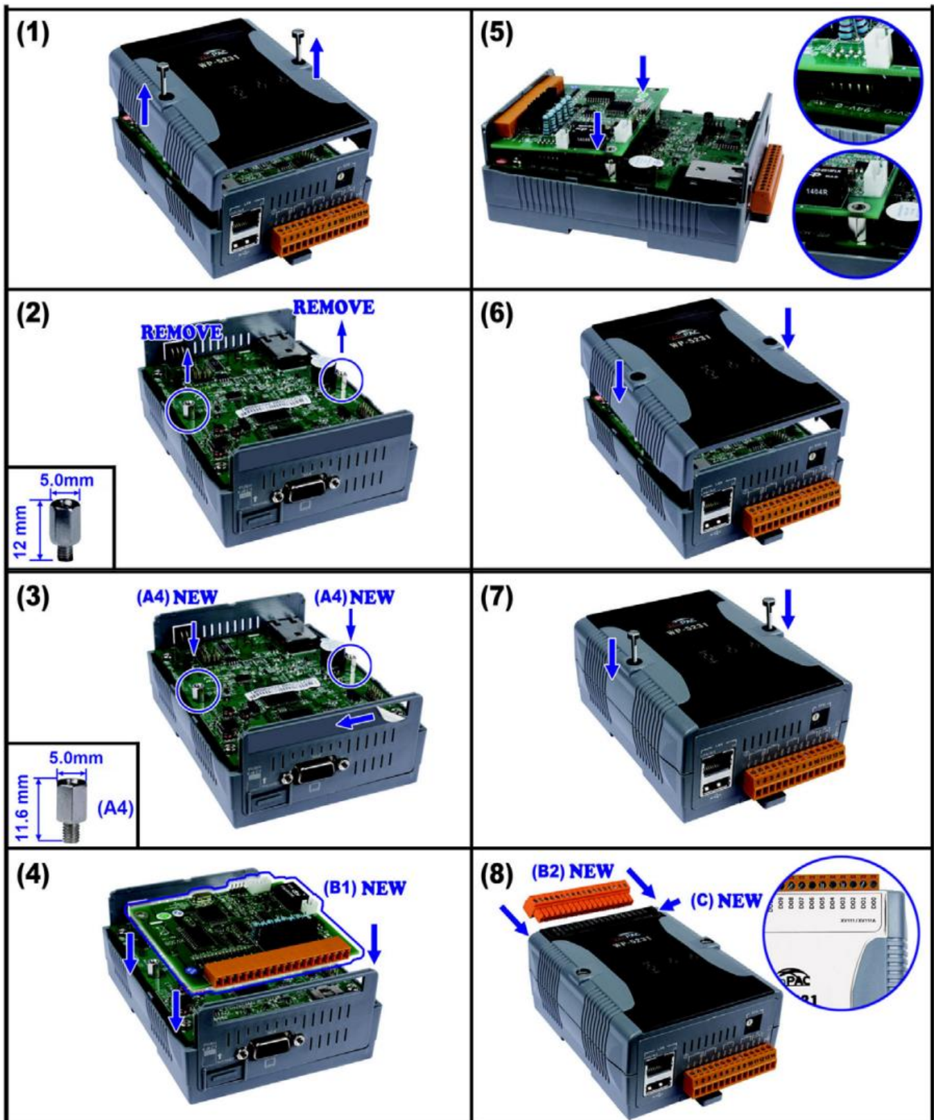
圖 288) 附錄 D.2 UA-5231 安裝 XV-board 步驟圖
