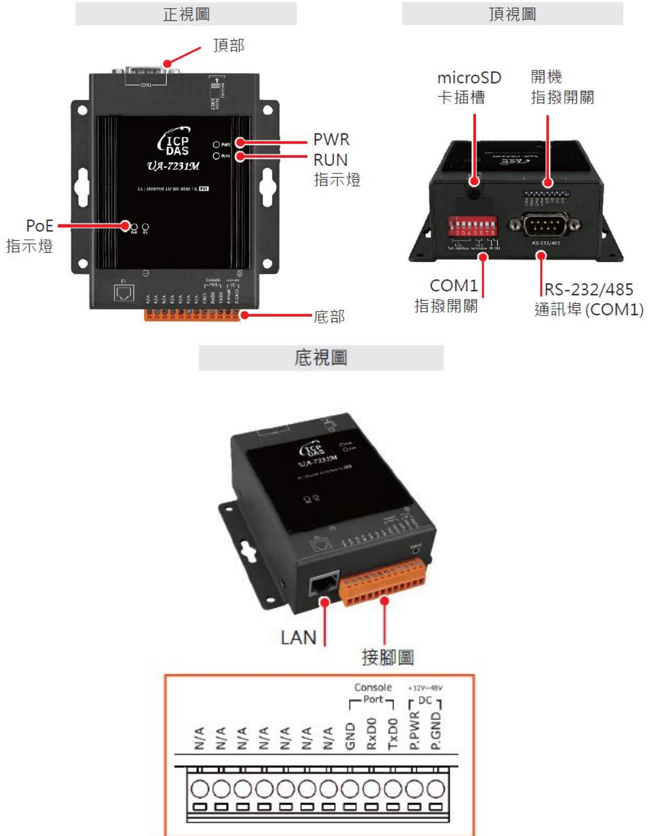
圖 5) 機構圖 UA-7231M
