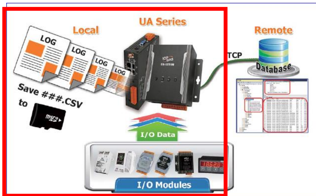
圖 248) 本地資料紀錄功能應用圖
