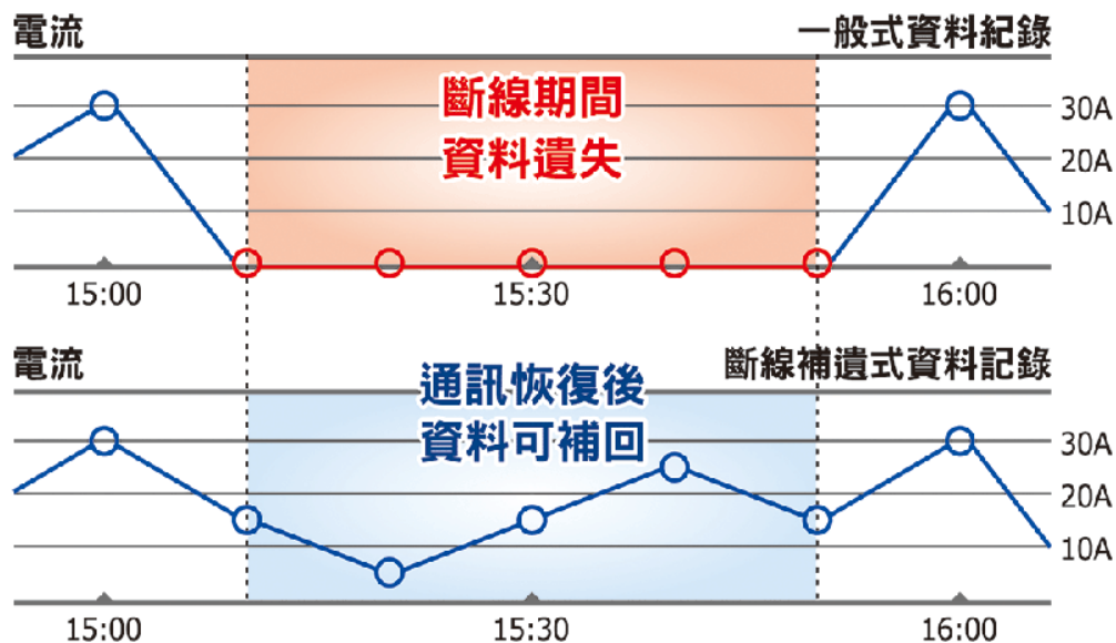
圖 294) 斷線補遺資料紀錄圖
