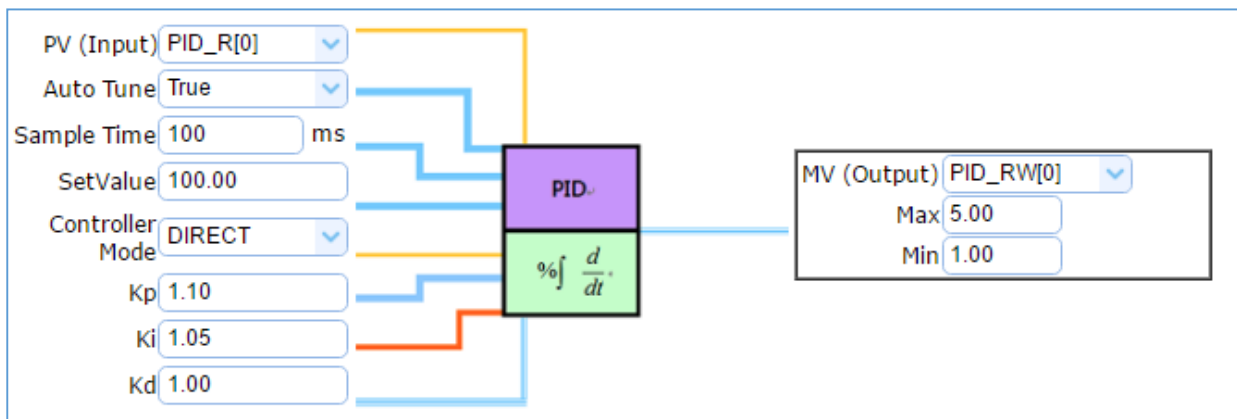
圖 213) PID 運算應用公式應用參考
