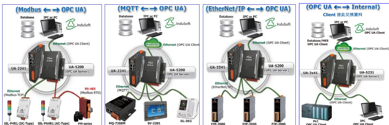
圖 156) 轉換功能區塊示意圖與應用方案架構圖
