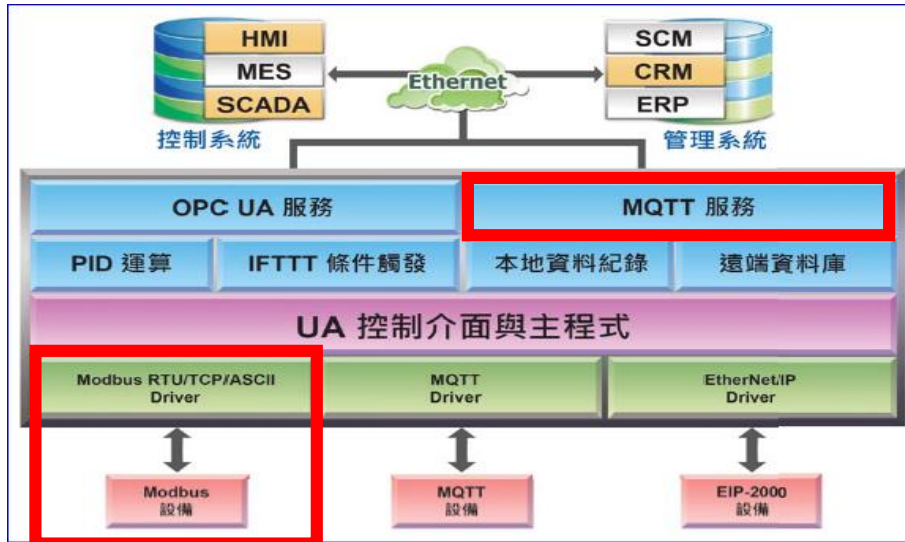
圖 197) MQTT JSON 和 Modbus TCP 轉換功能示意圖
