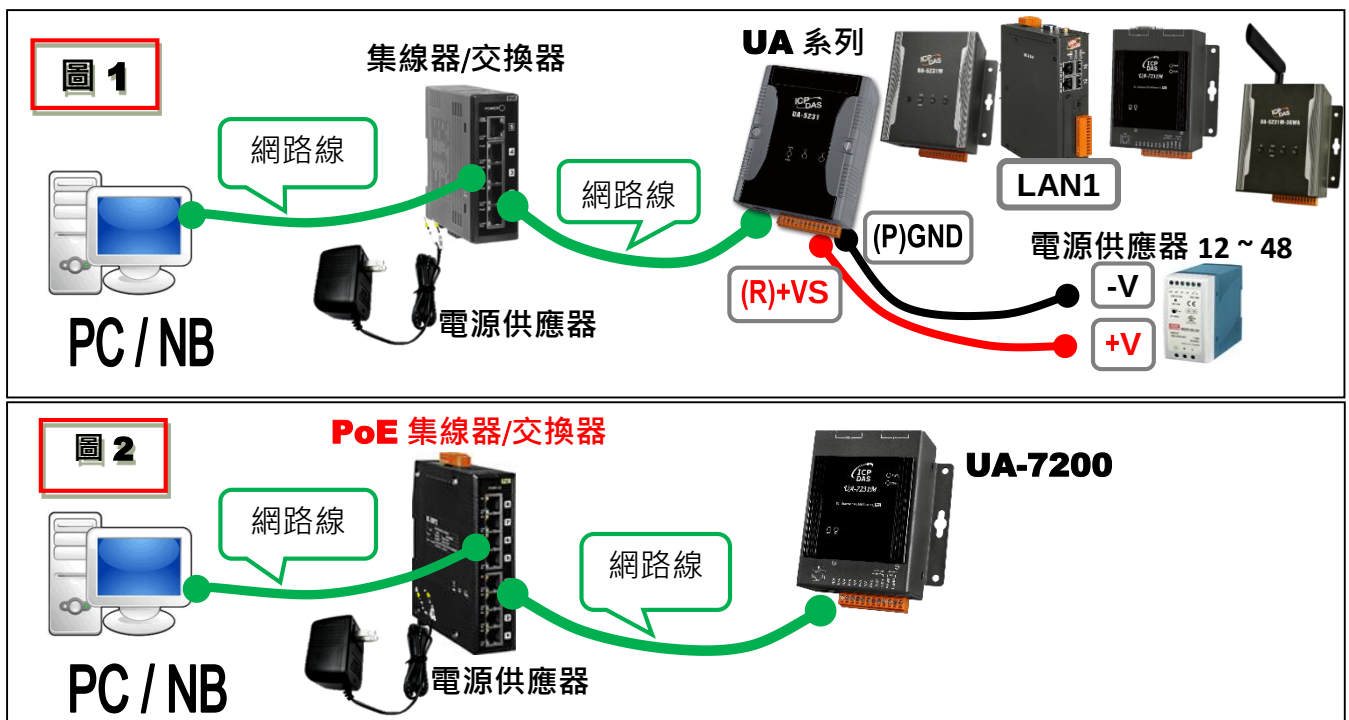
圖 14) CH2 硬體連接圖
