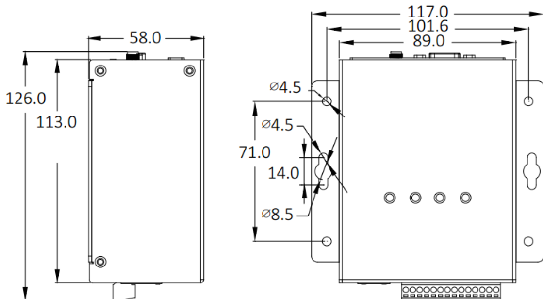
圖 12) 尺寸圖 UA-5200 系列
