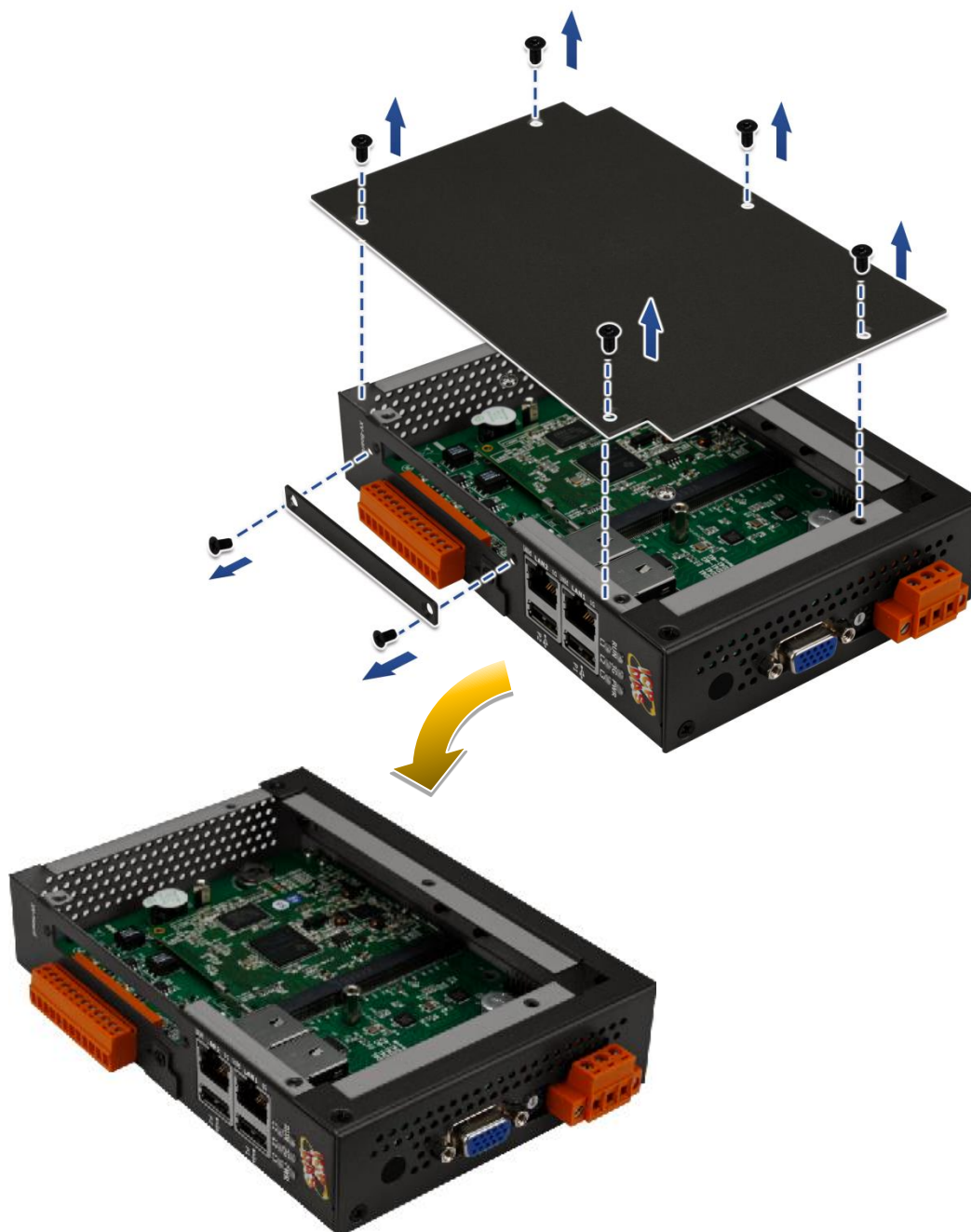
圖 284) 附錄 D.1 UA-2241M 安裝 XV-board 步驟 1
