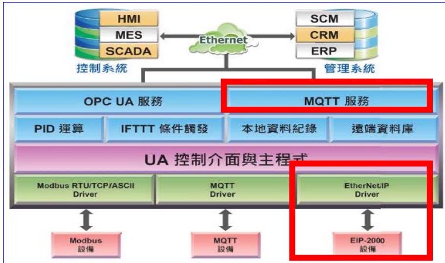
圖 188) MQTT 和 EtherNet/IP 轉換功能示意圖
