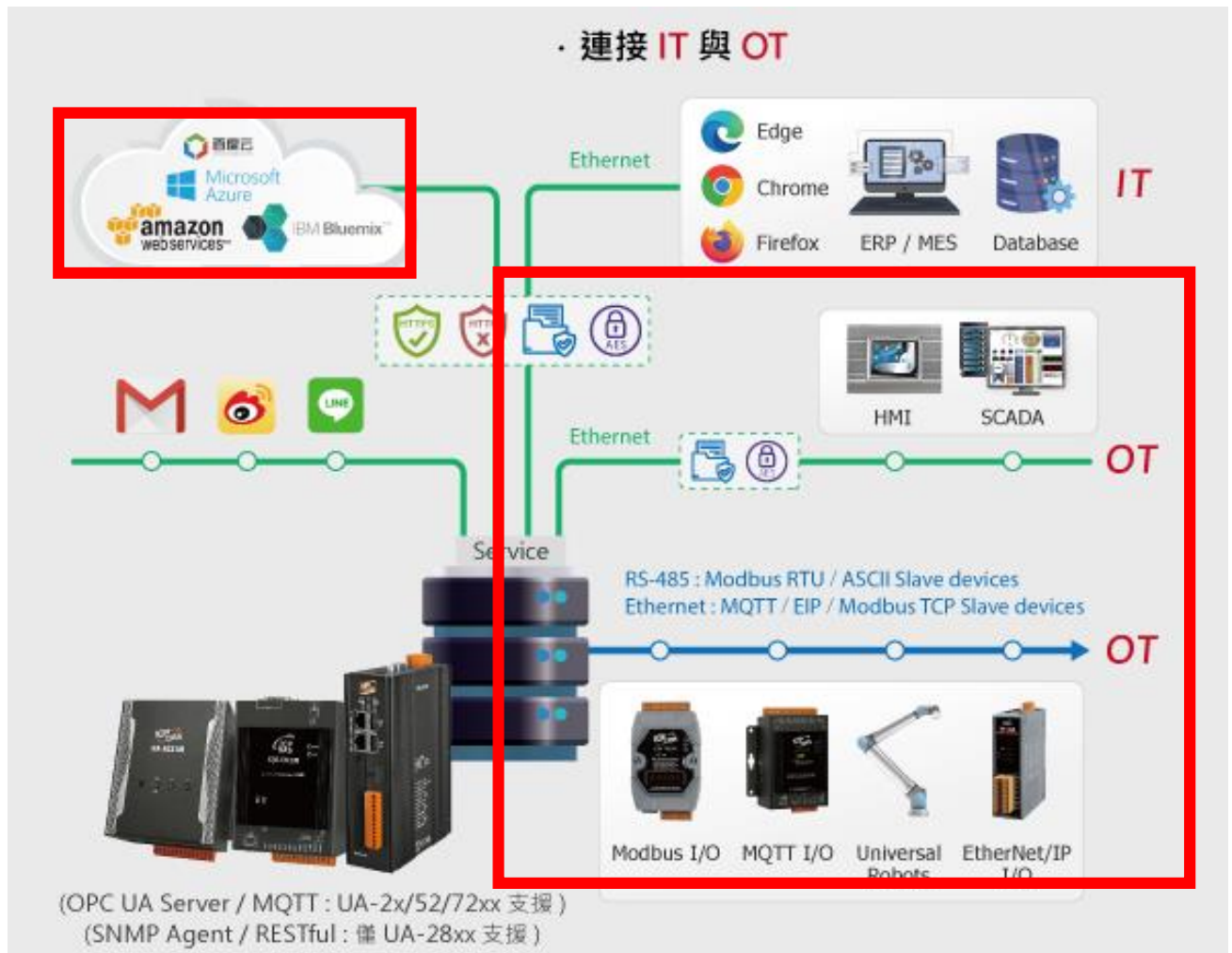
圖 136) MQTT 遠端 Broker 應用圖
