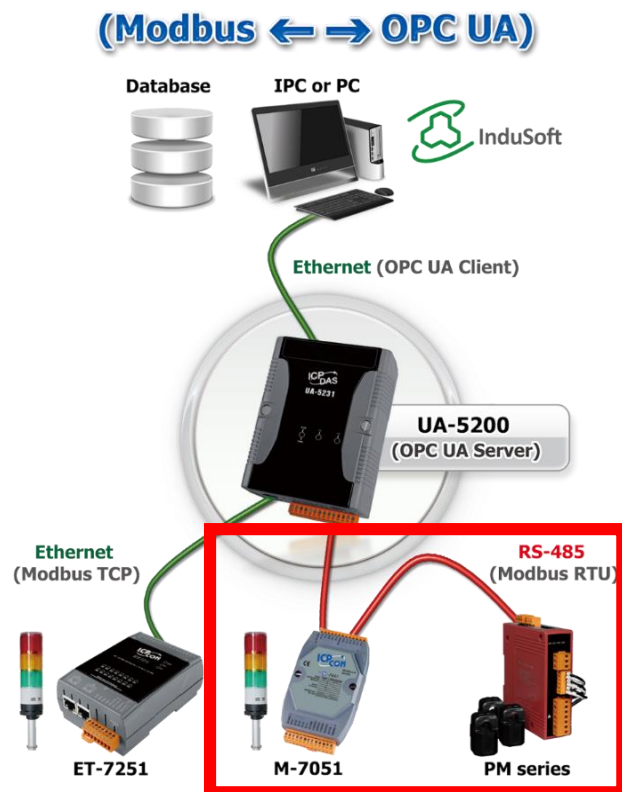
圖 158) OPC UA 和 Modbus 轉換功能應用方案架構圖
