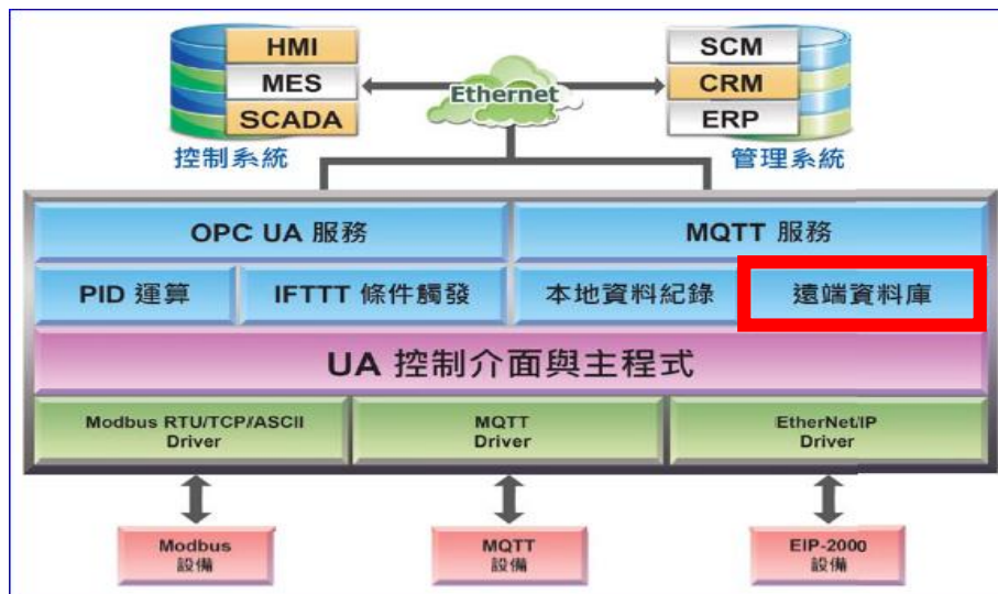
圖 235) 遠端資料庫功能示意圖
