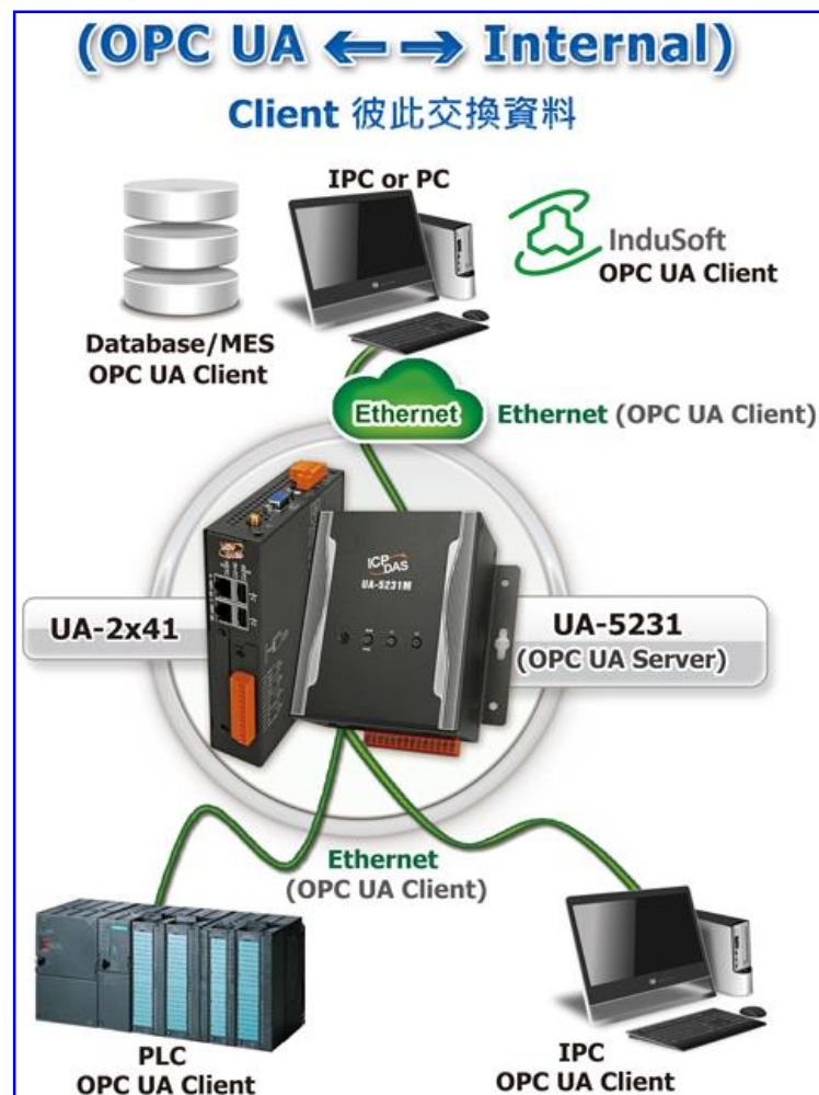
圖 175) OPC UA 和 Internal 轉換功能應用方案架構圖
