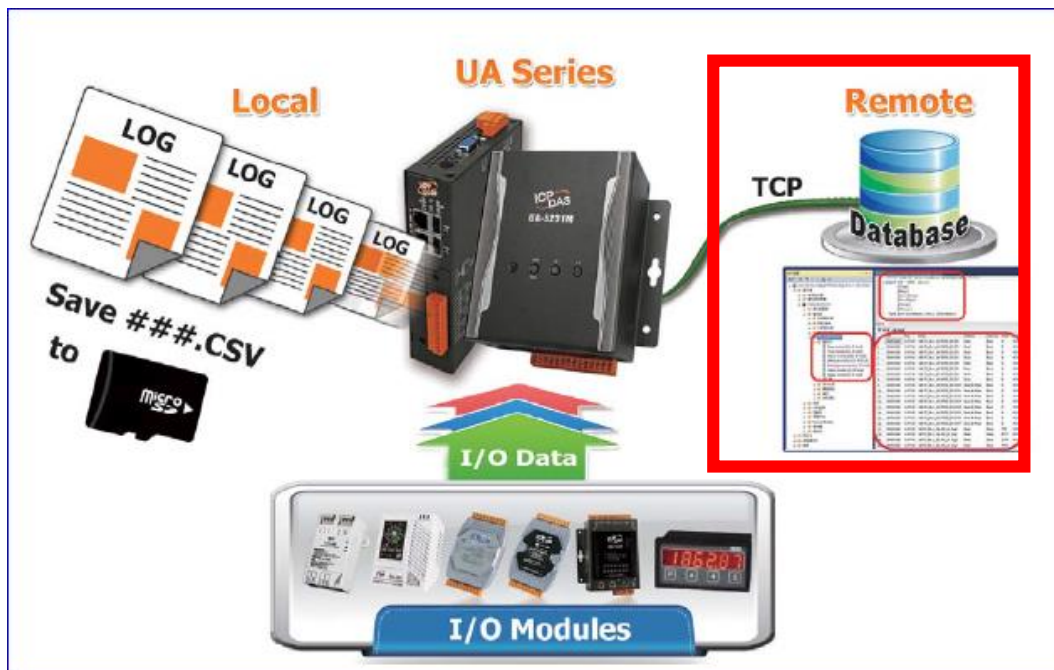
圖 229) 遠端資料庫應用圖
