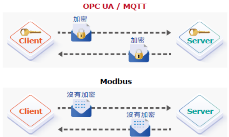
圖 264) MQTT 身分認證/資料加密功能
