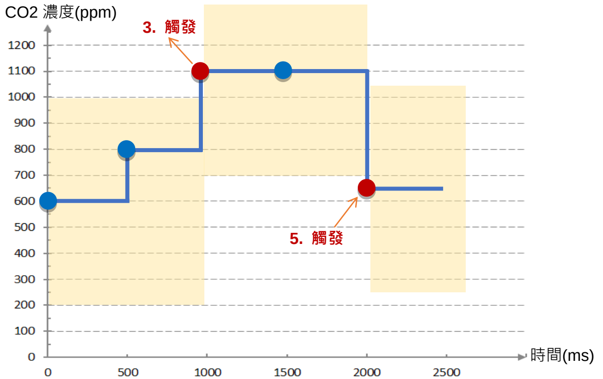
圖 221) 條件觸發方式說明圖：變數屬性 AIO
