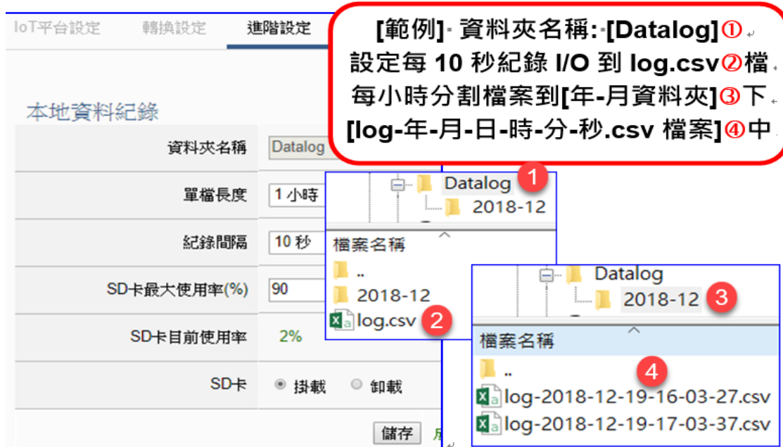
圖 227) 進階設定 > 資料紀錄器 - 本地資料紀錄器 設定步驟
