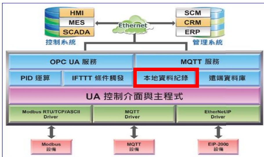
圖 224) 本地資料紀錄功能示意圖
