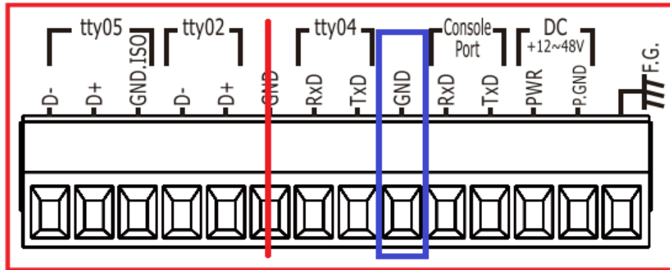
圖 8) 接腳圖 UA-5200 系列-2
