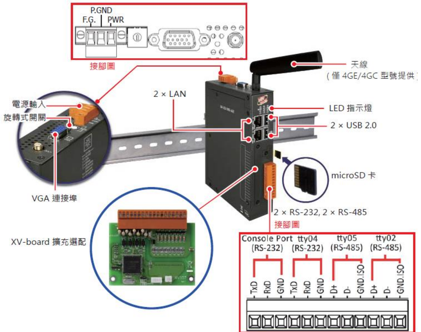
圖 1) CH1 機構圖 UA-2200 系列
