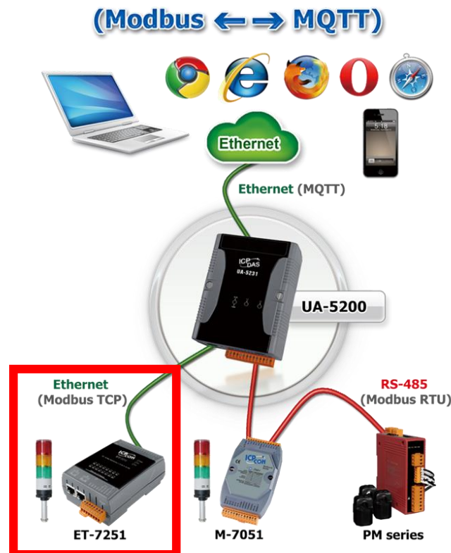
圖 198) MQTT JSON 和 Modbus TCP 轉換功能應用方案架構圖
